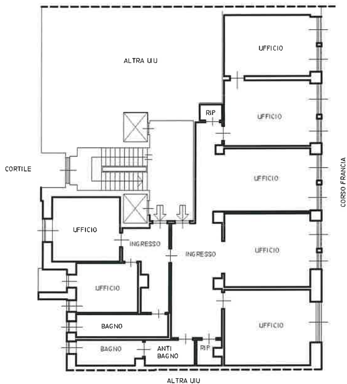
PIANTA PIANO SECONDO (3° F.T.) H. 3,00 M.
