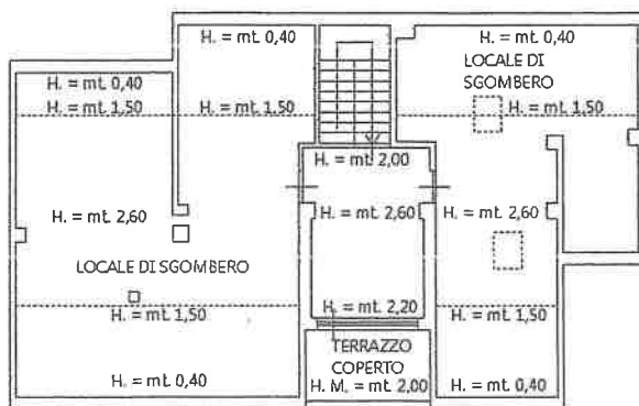
PIANO SECONDO (SOTTOTETTO)
